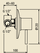
800034 __ __ Miscelatore monocomando incasso doccia, senza deviatore. Wall-mounted single lever shower mixer, without diverter.
