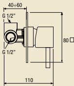
800039 __ Miscelatore monocomando incasso doccia, senza deviatore. Wall-mounted single lever shower mixer, without diverter.
