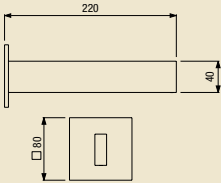
700018 __ Piantana a pavimento per riempimento vasca. Floor mounted bath mixer.
