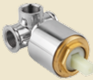
300028 __ Ø 40 Parte incasso comando doccia. Wall-mounted part for shower mixer.
