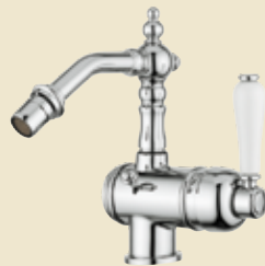
600019 _ _ Miscelatore monocomando bidet, flessibili inox G3/8", con scarico 1"1/4 con astina. Single lever bidet mixer, G3/8" stainless steel flexible hoses, with 1"1/4 pop-up waste.
