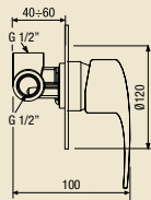
800043 __ Miscelatore monocomando incasso doccia, senza deviatore. Wall-mounted single lever shower mixer, without diverter.
