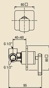
800026 __ Miscelatore monocomando incasso doccia, senza deviatore. Wall-mounted single lever shower mixer, without diverter.
