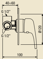
800050 _ _ Miscelatore monocomando incasso doccia, senza deviatore. Wall-mounted single lever shower mixer, without diverter.
