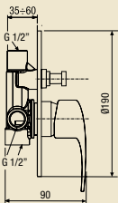
800044 __ Miscelatore monocomando incasso con deviatore. Wall-mounted single lever shower mixer, with diverter.
